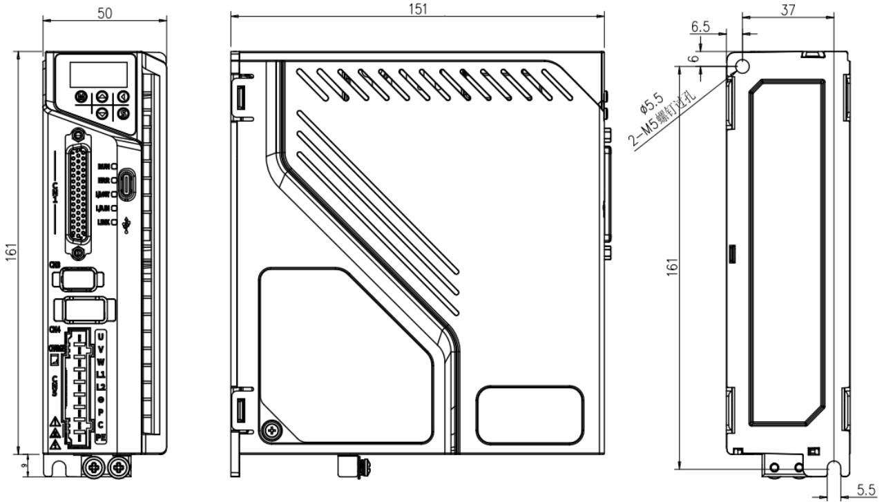
◆ SIZE-C 安装尺寸图 (单位 mm):
