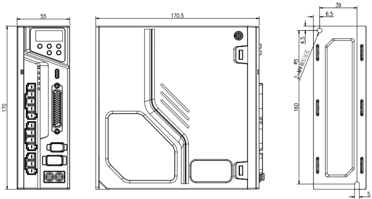
◆ SIZE-C 安装尺寸图 (单位 mm):
